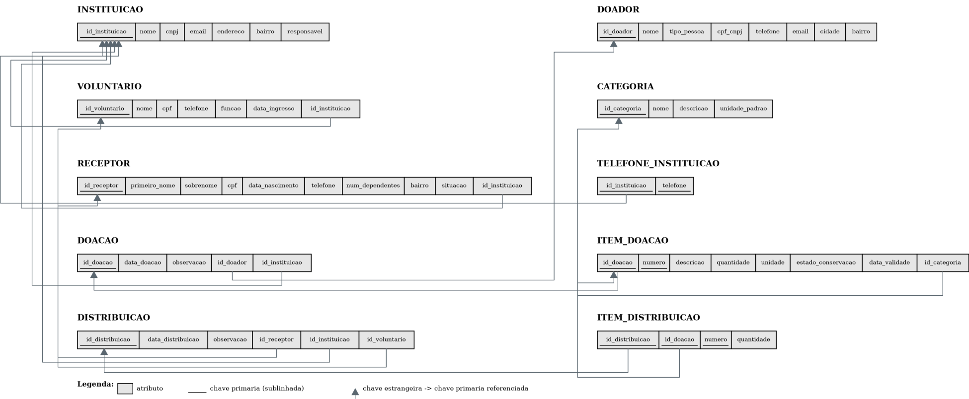
Modelo Logico - Diagrama de Esquema Sistema de Doacoes - ONG "Somos do BHem"
