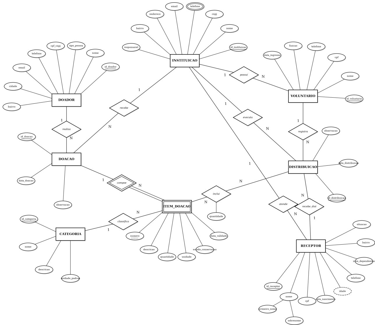
Modelo Conceitual - Diagrama Entidade-Relacionamento (Notação Peter Chen) Sistema de Doacoes - ONG "Somos do BHem"
